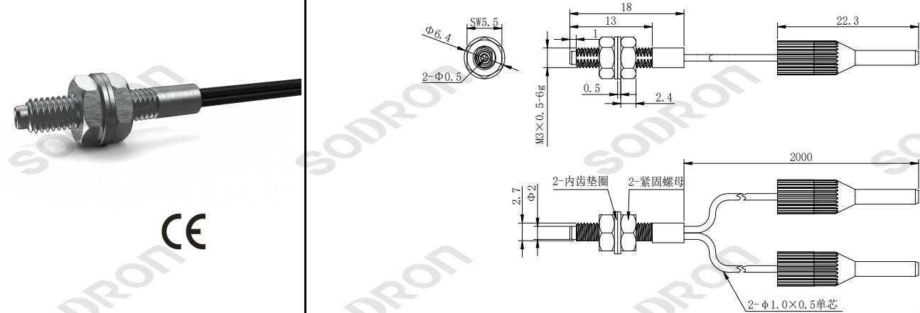
外形尺寸图
