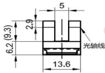
端子配置
