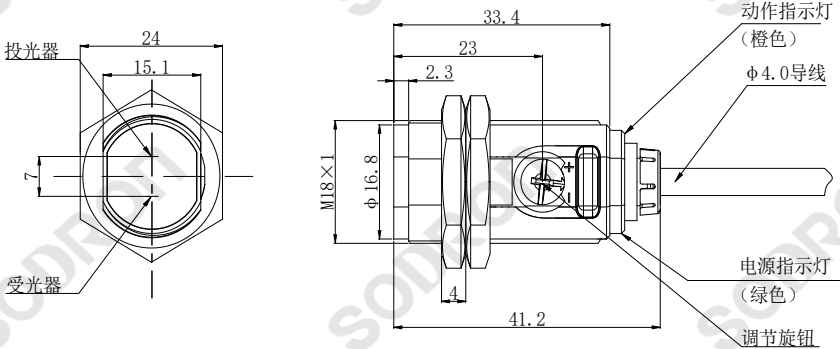
外形尺寸图
