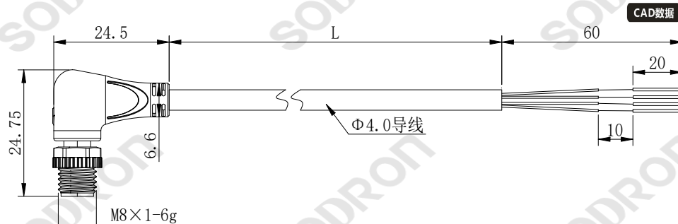
外形尺寸图
