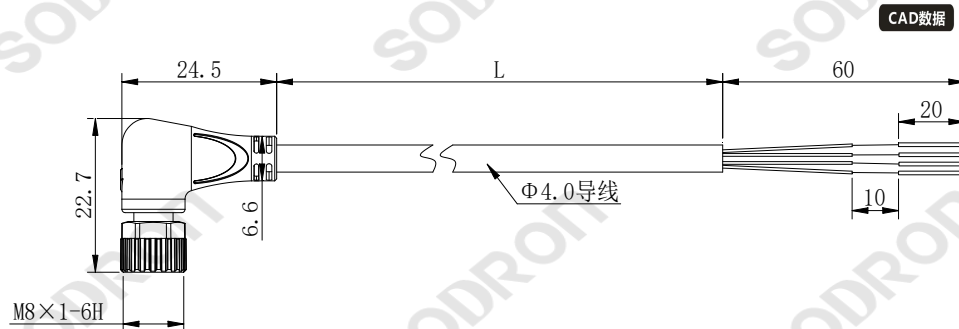
外形尺寸图
