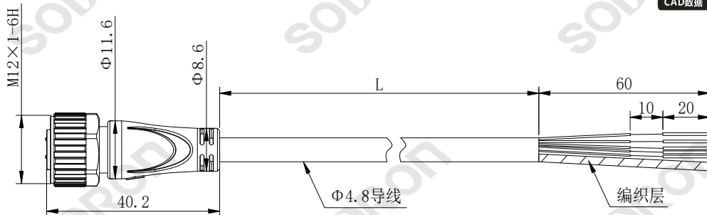
外形尺寸图
