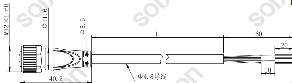
外形尺寸图
