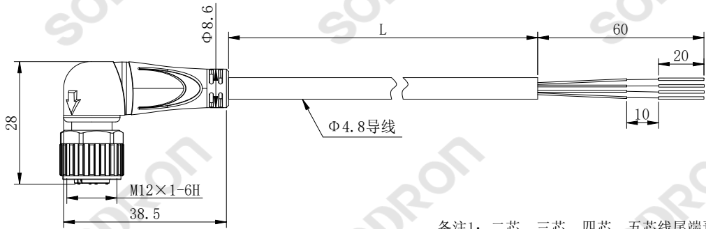
外形尺寸图
