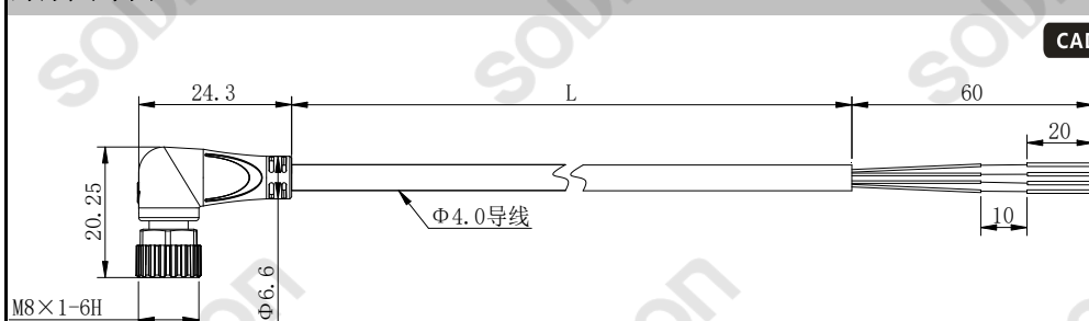
外形尺寸图
