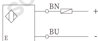
接线方式
