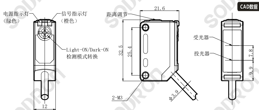
外形尺寸图
