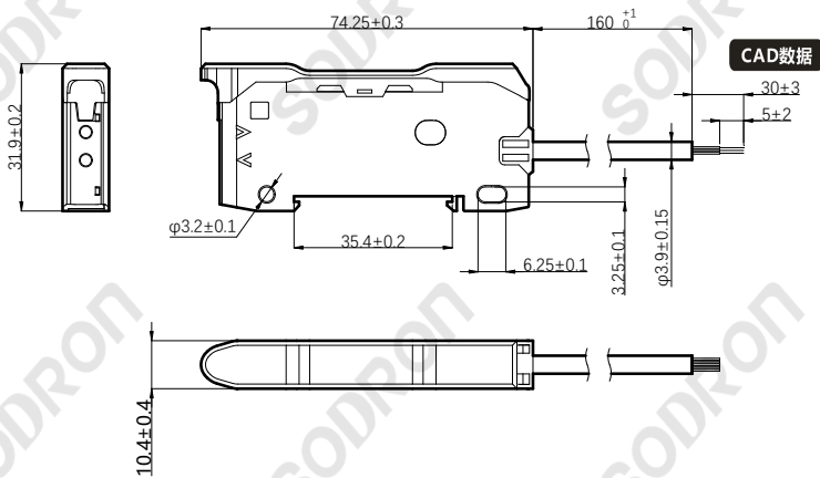
外形尺寸图
